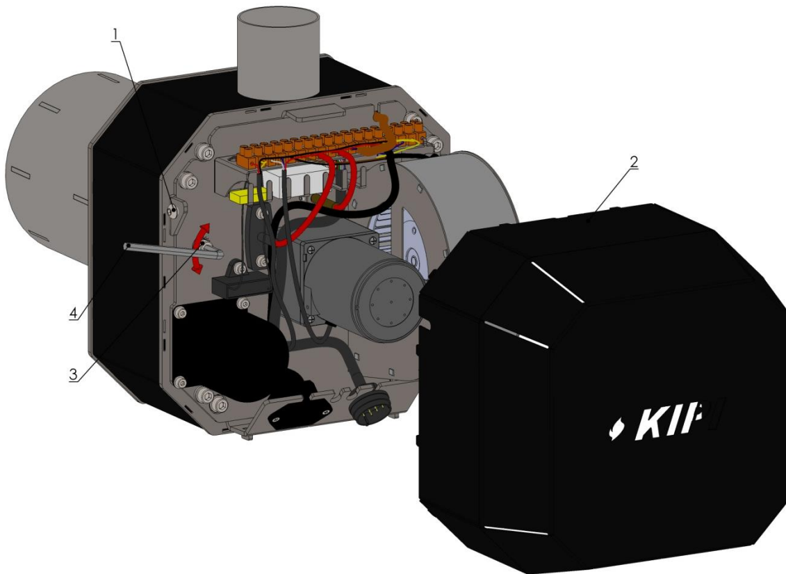
Рис. 7. Регулювання подачі повітря в камеру спалювання.
